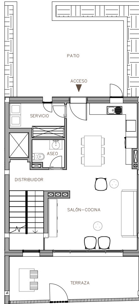
PLANTA BAJA
