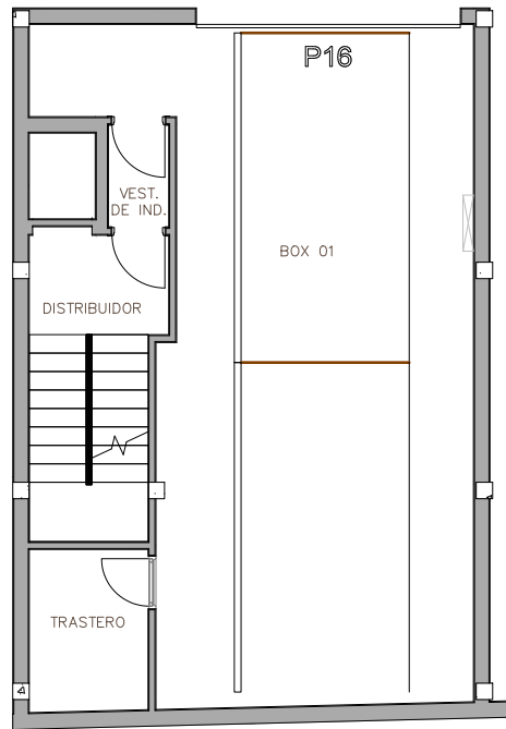
PLANTA SOTANO
