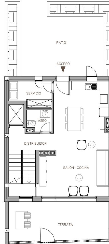
PLANTA BAJA
