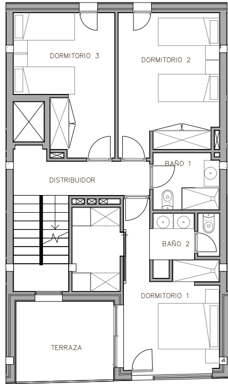
PLANTA PRIMERA
