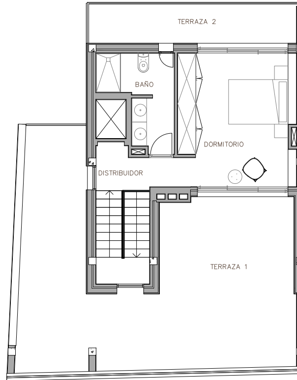
PLANTA SEGUNDA
