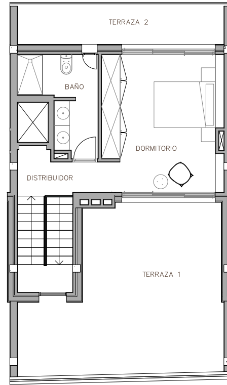
PLANTA SEGUNDA
