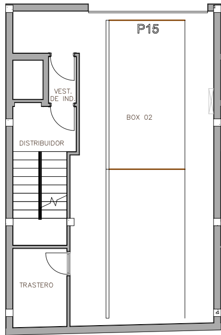
PLANTA SOTANO
