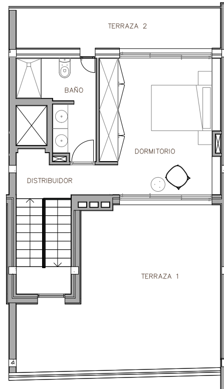
PLANTA SEGUNDA
